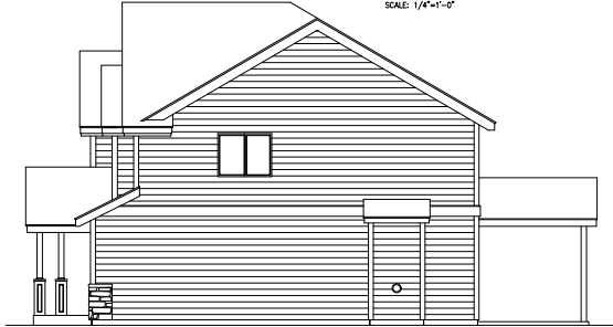
RIGHT ELEVATION SCALE: 1/4"=1'-0"
